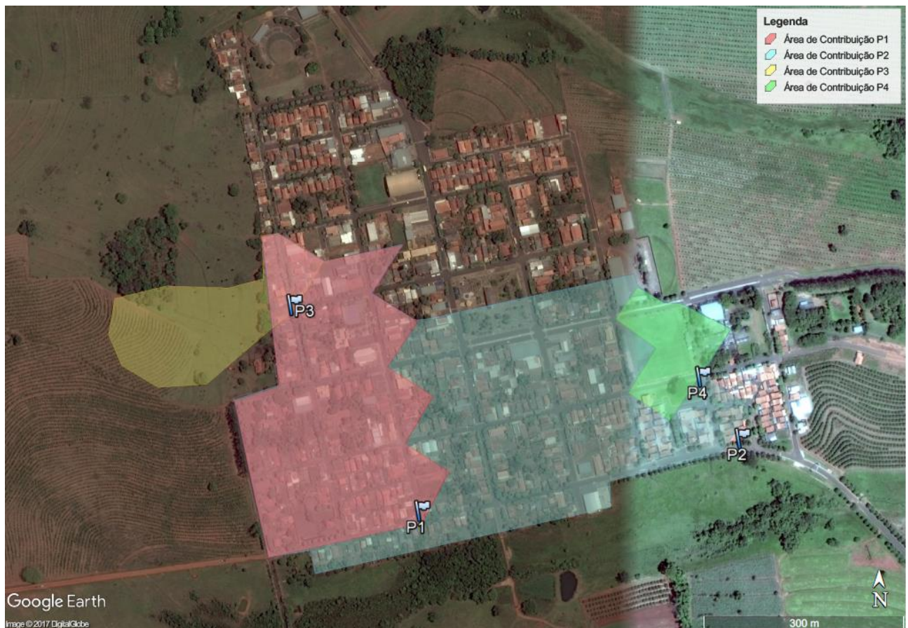
Figura 4.1 – Pontos críticos do sistema de drenagem
