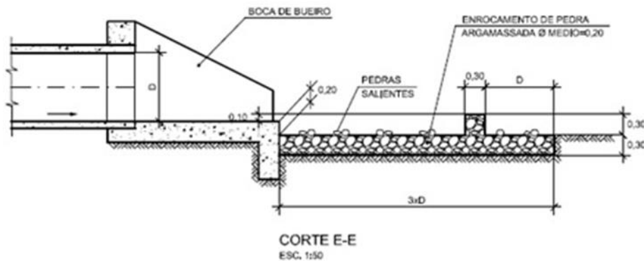
Ilustração 8.5 – Dissipador
