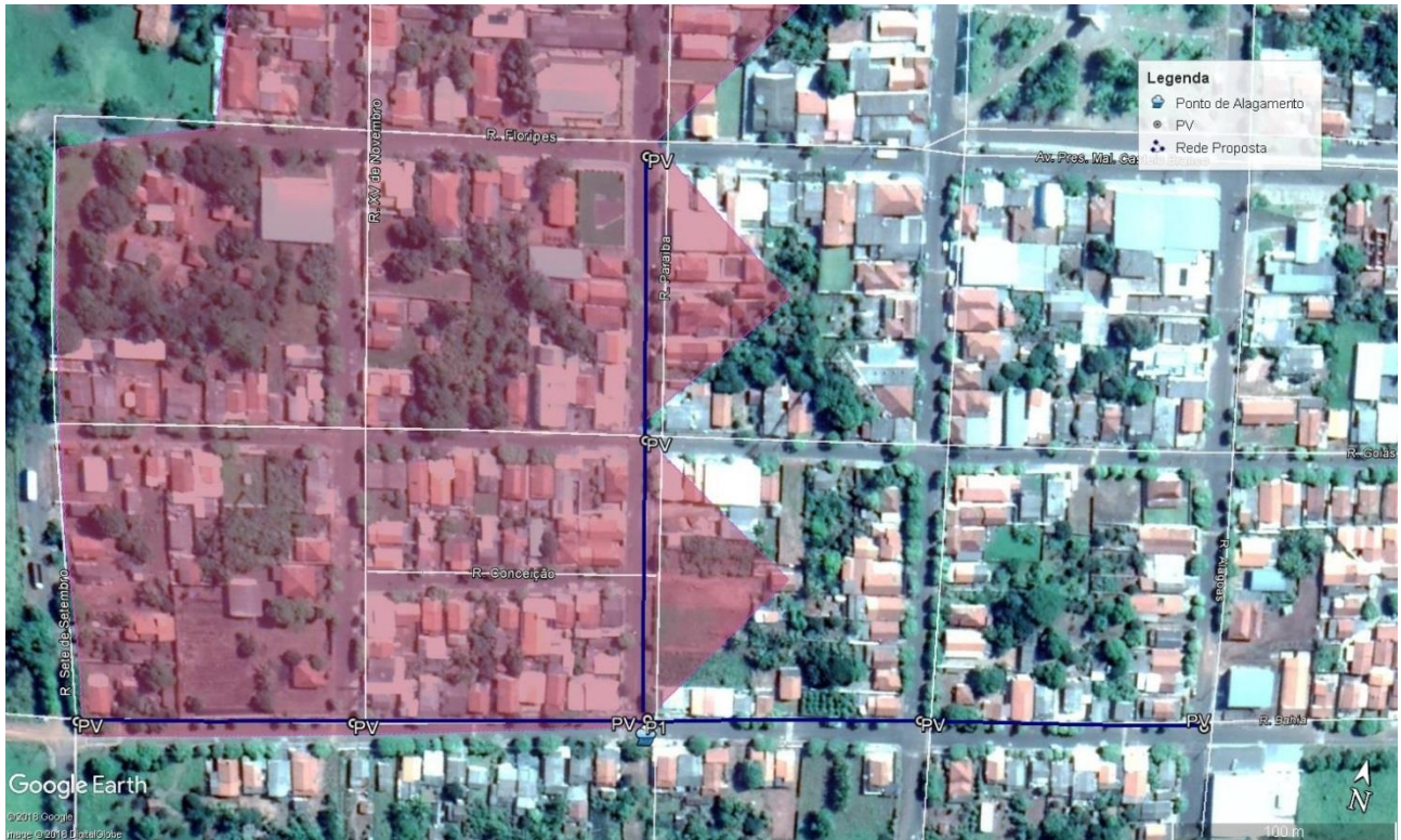
Ilustração 8.1 – Intervenções Propostas para o Ponto de Alagamento 1
